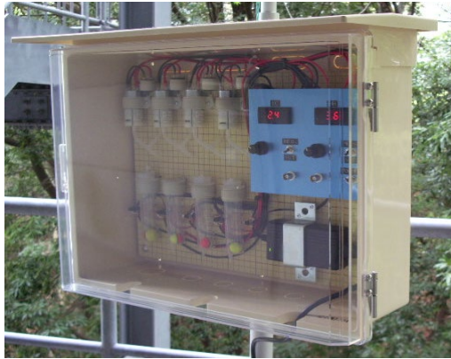
水耕栽培 (液肥コントローラ)
